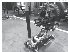
プレーキドラム脱着サポート治具
