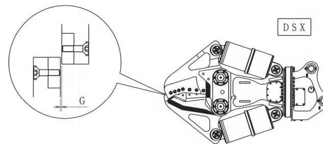
図 6-2 カッターの隙間測定
