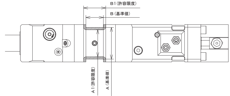
図 7-1-6 ブラケット溝測定部位 ( PH-06 ~ PH-4 )
