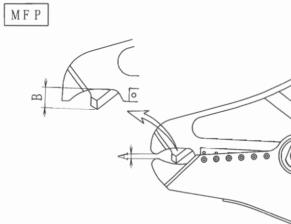
図 6-6 先端ポイント・圧砕ポイントの測定
