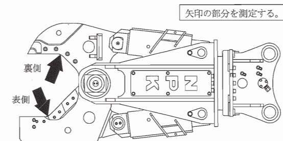
図 7-13 カッターの隙間測定位置
