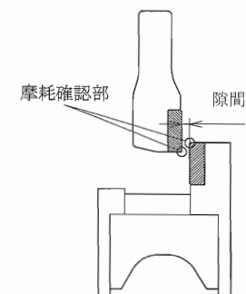
図 7-2 カッターの隙間測定
