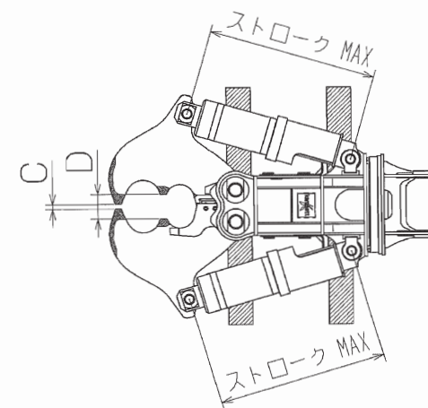
図 4-15 圧砕ポイントの測定
