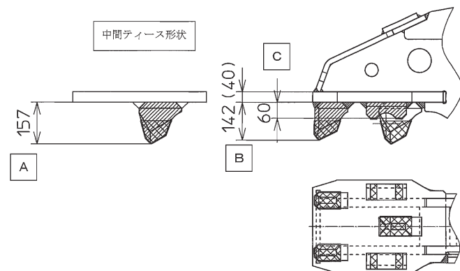
(7) 型式 G-175
