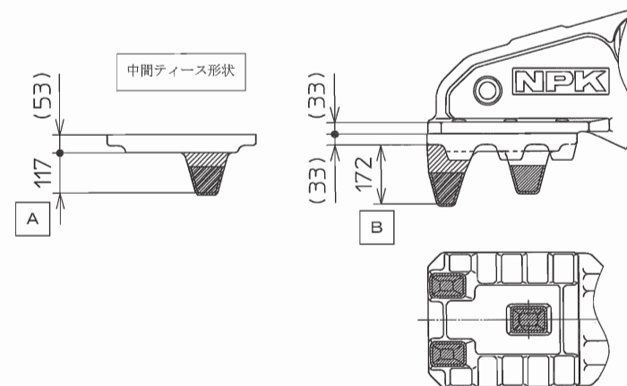
(8) 型式 G-200
