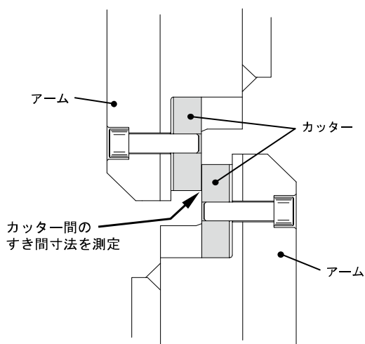
図7-1-3 カッタすき間の測定箇所(断面図)
