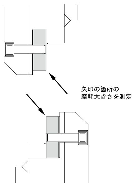
図7-1-4 カッタ摩耗限度の測定箇所(断面図)
