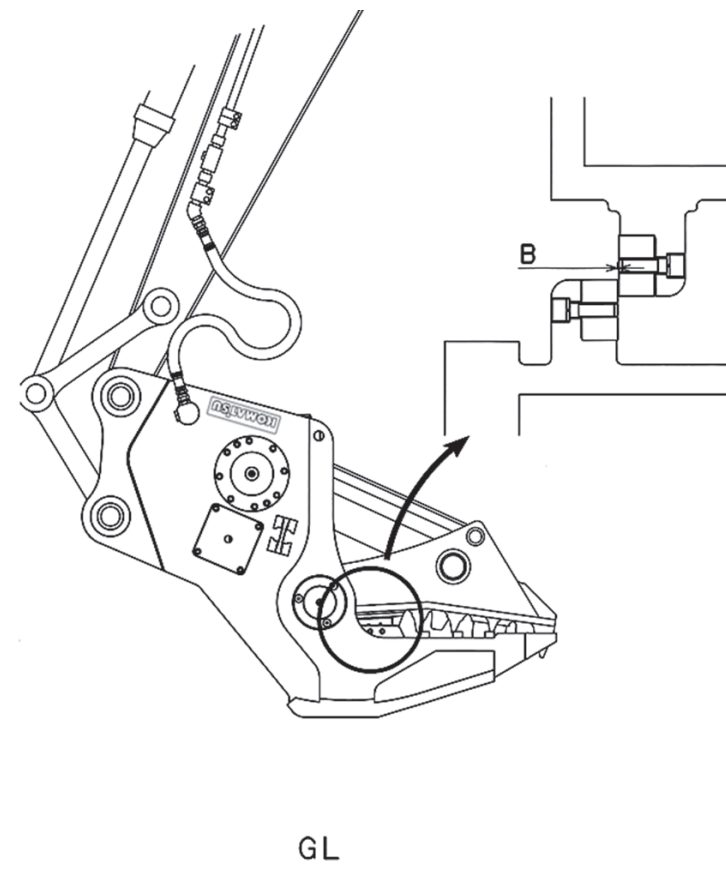
図 1-13 カッターのすき間測定
