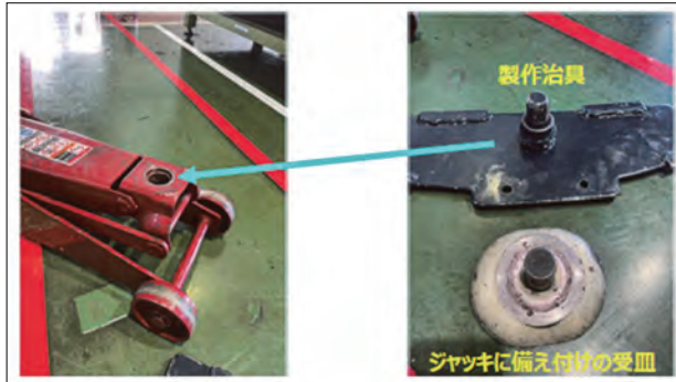
ガレージジャッキ受け皿のボス穴を利用し、 考案した治具を取り付け
