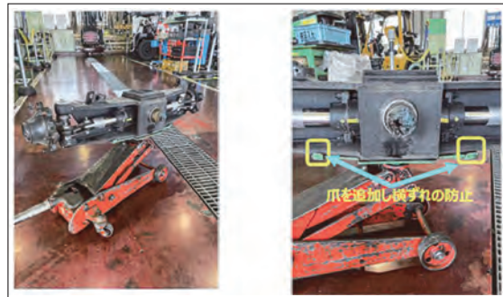
リヤークスル搭載状況 (横ずれ防止の爪で落下防止対策)
